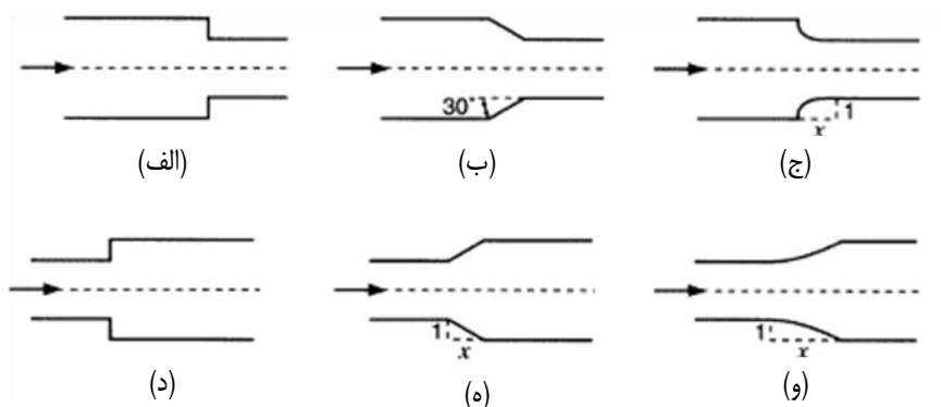
شکل ۲۲- مبدلهایی با طراحی مختلف (الف) انقباض بدون وجود مبدل (ب) انقباض با وجود مبدل پخ خورده مستقیم (ج) انقباض با وجود مبدل ماهیچه‌ای شکل (د) انبساط بدون وجود مبدل (ه) انبساط با وجود مبدل پخ خورده مستقیم (و) انبساط با وجود مبدل ماهیچه‌ای شکل.
