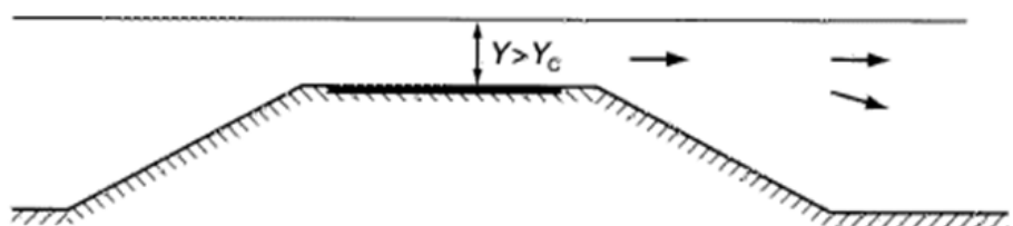
جریان مستغرق (د)
