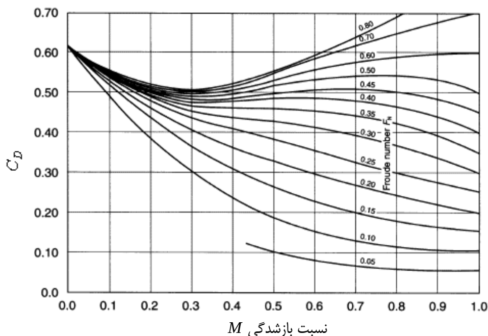
شکل ۱۳- نمودار ضریب C_D در برابر نسبت بازشدگی M
