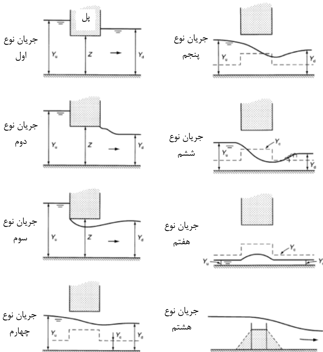
شکل ۴- طبقه‌بندی انواع جریان عبوری از محل پل
