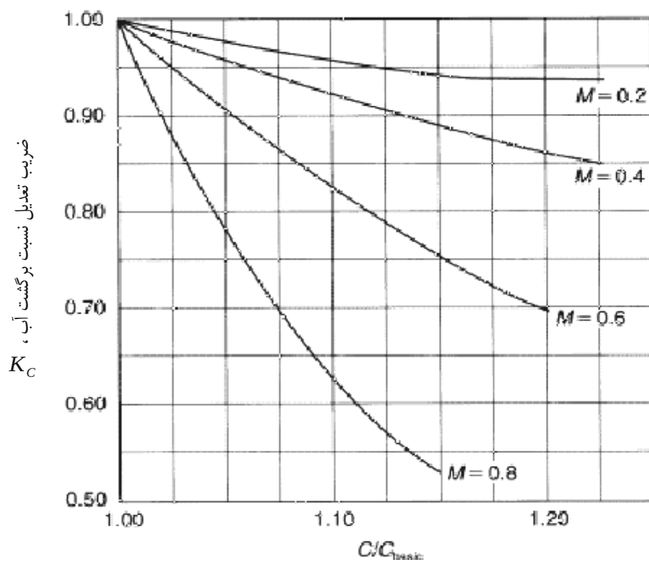
شکل ۷- تعیین ضریب K_c در روش USGS
