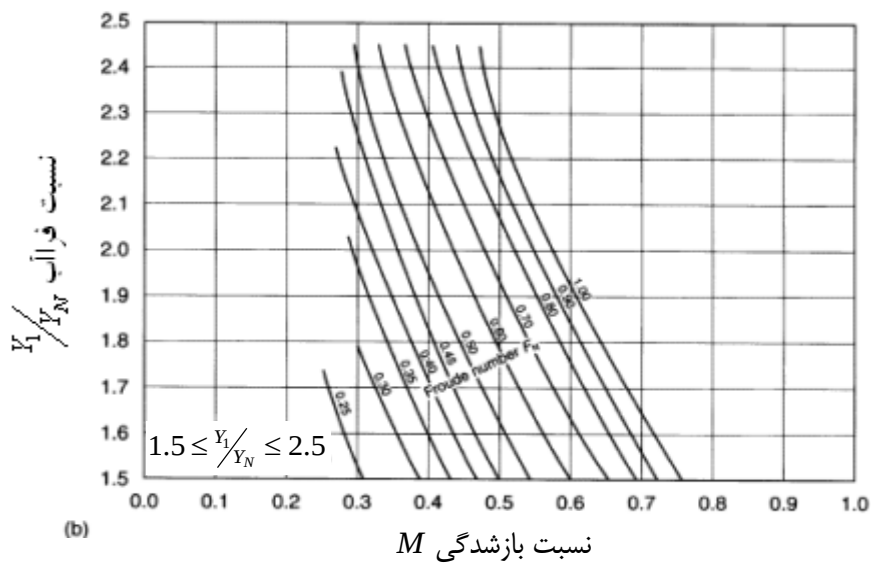
شکل ۱۰- منحنی تغییرات Y_1/Y_N در مقابل نسبت بازدهی M و عدد فرود عمق نرمال Fr_N
