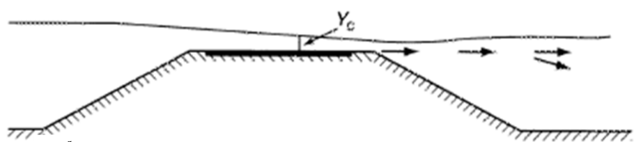
جریان سطحی آزاد (ب)
