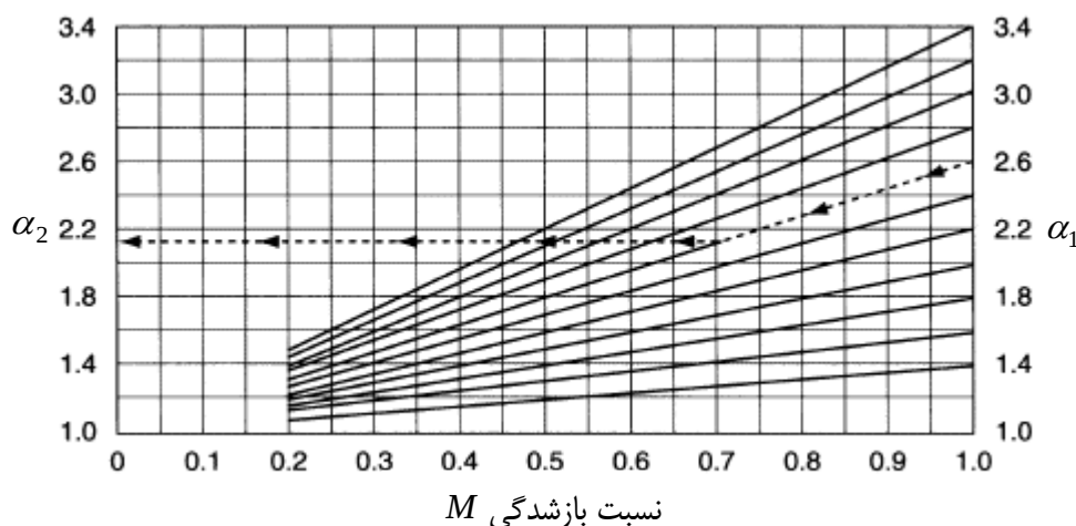
شکل ۸- محاسبه \alpha_2 با استفاده از مقادیر \alpha_1 و نسبت بازشدگی M
