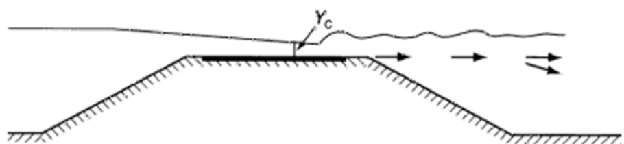
جریان سطحی آزاد مشرف به جریان مستغرق (ج)
