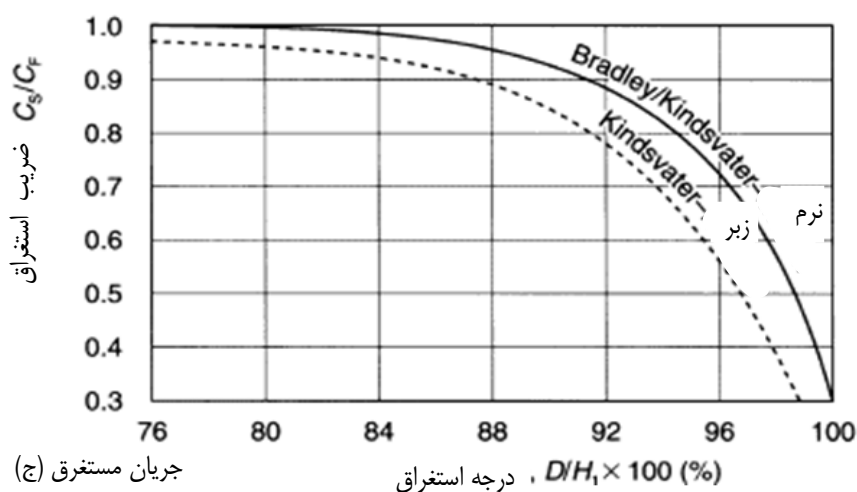
شکل ۲۰- ضرایب دبی برای خاکریزها (الف) و (ب) برای جریان آزاد و (ج) برای جریان مستغرق
