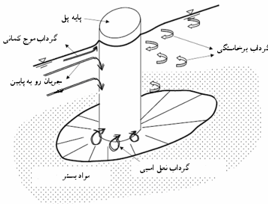
شکل ۳۳- جریان و الگوی آبشستگی در اطراف پایه استوانه‌ای شکل
