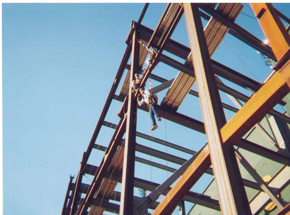
شکل ۲-۱- جلوگیری از سقوط فرد با استفاده از کمربند ایمنی
